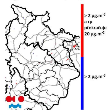
PM 2,5 - oblasti s příspěvkem > 2 \mu\text{g}\cdot\text{m}^{-3} primární PM 2,5 z REZZO 1 a 2 - průmysl
