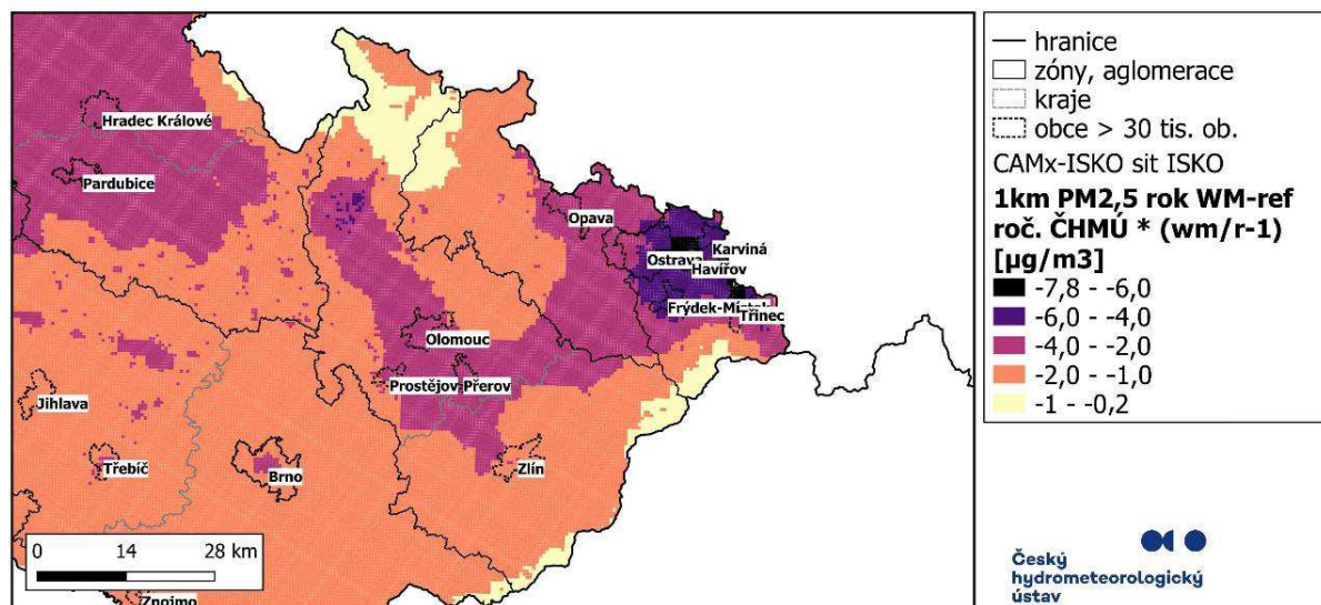
Obr. 66: Rozdíl ročních imisních koncentrací částic PM 2,5 mezi výhledovým rokem 2023 a výchozím rokem 2015 (na základě mapy ČHMÚ), zóna CZ07
