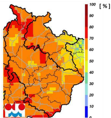
PM 2,5 - příspěvek k ročnímu průměru sekundární částice
