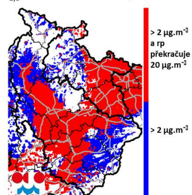
PM 2,5 - oblasti s příspěvkem > 2 \mu\text{g}\cdot\text{m}^{-3} primární PM 2,5 z REZZO 3 - lokální vytápění
