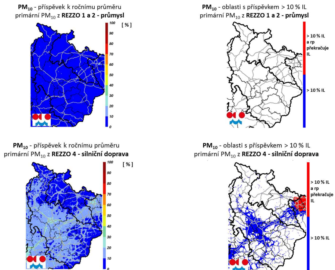
Obr. 33: Příspěvek primárních částic z českých zdrojů (průmysl a silniční doprava) k ročnímu průměru PM 10 – zóna CZ07
