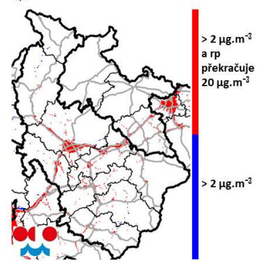
PM 2,5 - oblasti s příspěvkem > 2 \mu\text{g}\cdot\text{m}^{-3} primární PM 2,5 z REZZO 4 - silniční doprava
