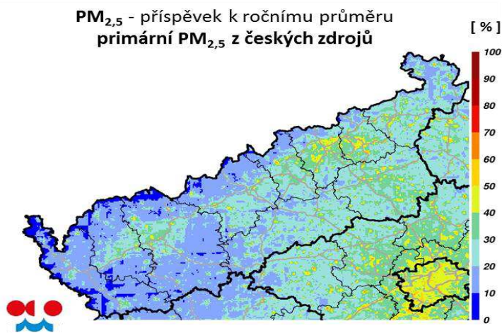
Obr. 36: Příspěvek sekundárních částic a primárních částic ze zahraničí, resp. primárních částic z českých zdrojů k ročnímu průměru PM 2,5 – zóna CZ04
