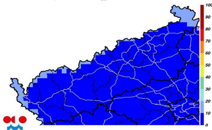
PM 10 - příspěvek k ročnímu průměru primární PM 10 ze zahraničí
