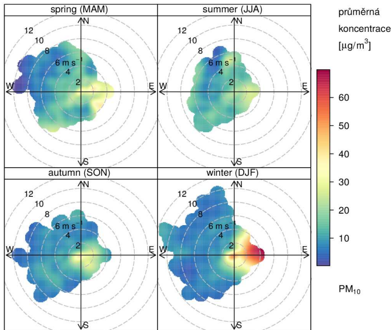
Obr. 84: Sezónní koncentrační růžice pro PM 10 , zóna CZ04, stanice UTPM, 2011–2016
